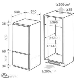
Einbauskizze zu EKGC225-40-110F
