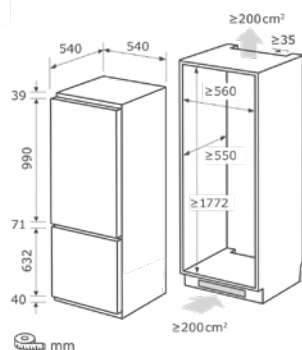
Einbauskizze zu EKGC270-70-NF-010E
