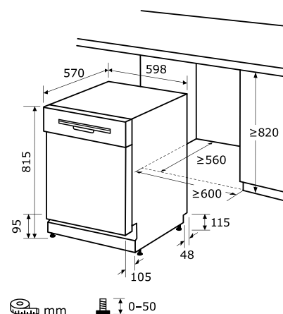
Einbauskizze zu EGSP6112-EF-030E inox
