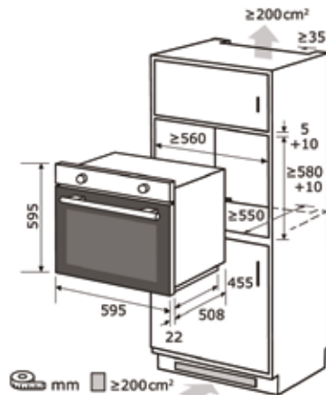
Einbauskizze zu EBE 657-2 Hsw
