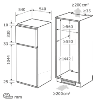
Einbauskizze zu EKGC265-40-040E
