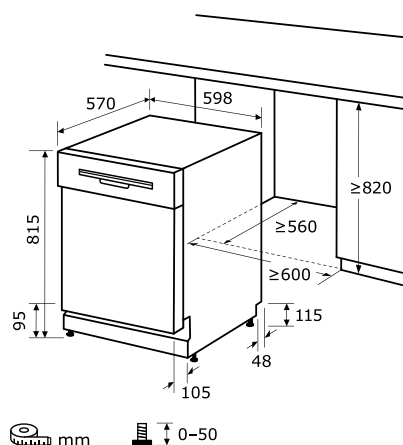
Einbauskizze zu EGSP9414-EF-030D inox
