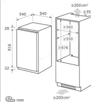
Einbauskizze zu EKS131-3-040F
