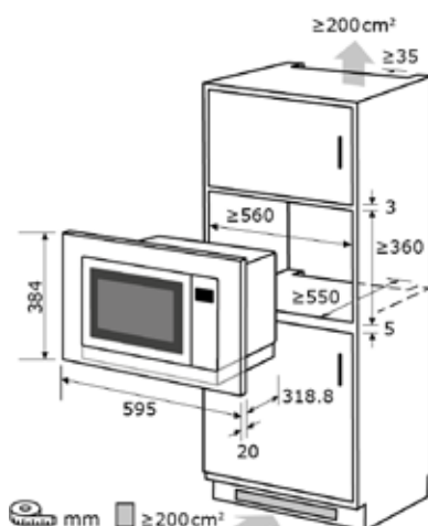
Einbauskizze zu EMW10-020 schwarz | inox
