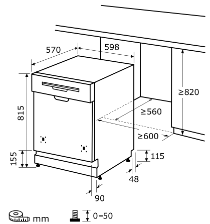
Einbauskizze zu EGSP2113-EB-030E inox
