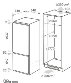
Einbauskizze zu EKGC270-70-E-040E
