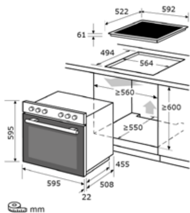
Einbauskizze zu EHE157-2UR-Set
