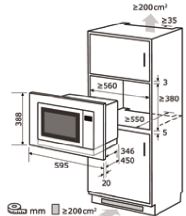
Einbauskizze zu EMW 2539.1 HI
