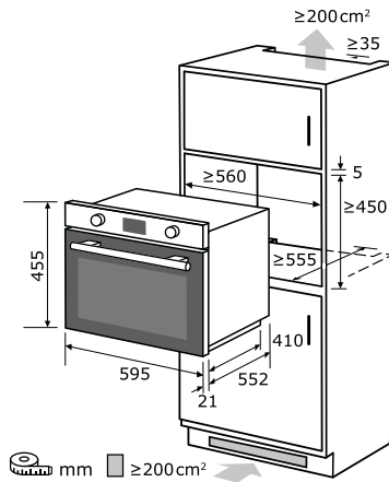
Einbauskizze zu EBM 4544 HI
