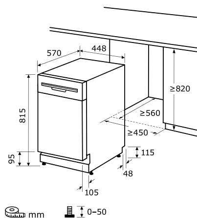
Einbauskizze zu EGSP9309-EF-030E inox
