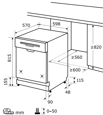
Einbauskizze zu EGSP1012-EB-030E inox
