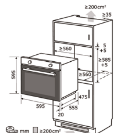
Einbauskizze zu EBEP 697-3 H
