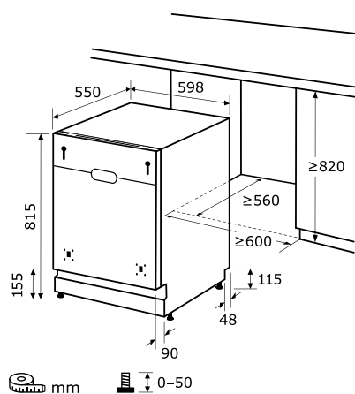
Einbauskizze zu EGSP9414-E-030D inox
