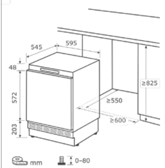
Einbauskizze zu UKS130-4-FE-010E
