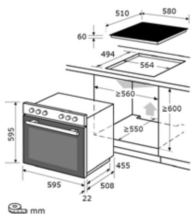
Einbauskizze zu EHE146-2.1-Set
