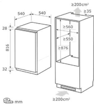
Einbauskizze zu EKS131-V-040F
