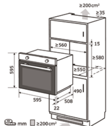
Einbauskizze zu EBE 555-1.2 U
