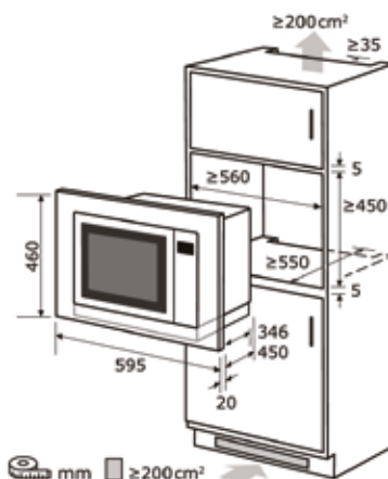
Einbauskizze zu EMW 2546.1 HI
