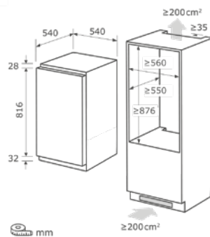
Einbauskizze zu EKS131-3-040E
