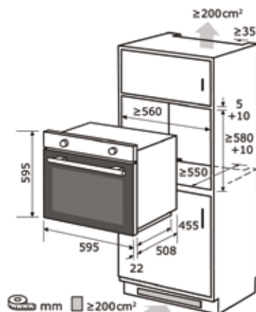
Einbauskizze zu EBE 657-2 U | EBE 657-U-020 schwarz
