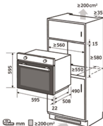
Einbauskizze zu EBE 65-1 H
