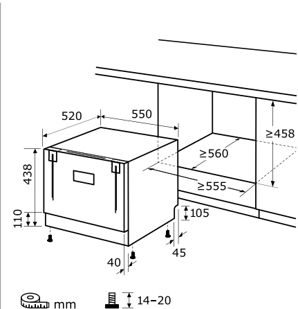
Einbauskizze zu EGSP1060-E-030F schwarz
