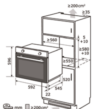
Einbauskizze zu EBEP 707-18 H
