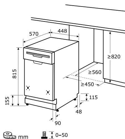
Einbauskizze zu EGSP9410-EB-030D inox
