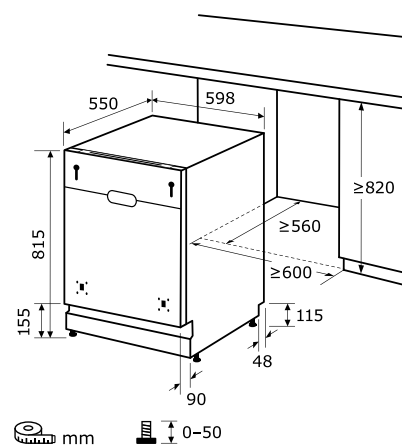
Einbauskizze zu EGSP6312-E-030D silber | EGSP6012-E-030E silber
