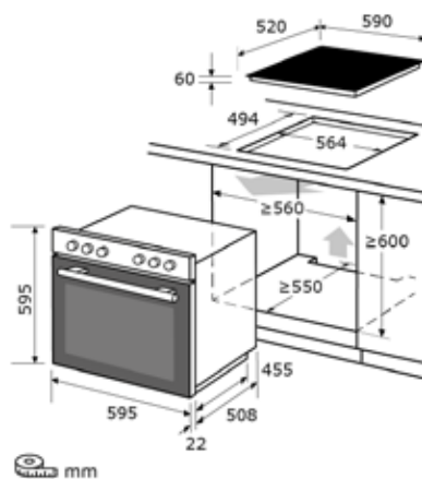
Einbauskizze zu EHE 156-2.IUBZ-Set
