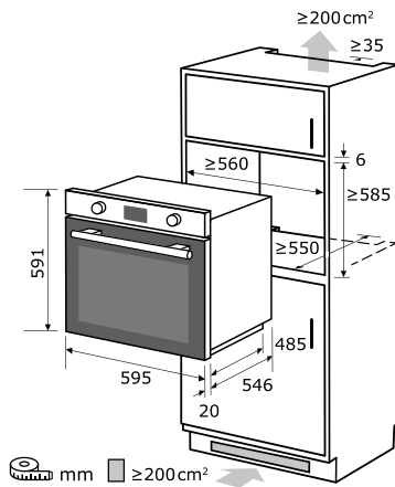
Einbauskizze zu EBEM 797-H-030 schwarz
