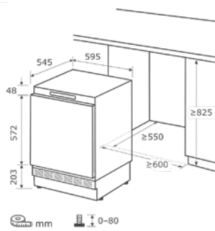
Einbauskizze zu UKS130-4-FE-010F
