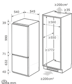
Einbauskizze zu EKGC270-70-NF-F-010E
