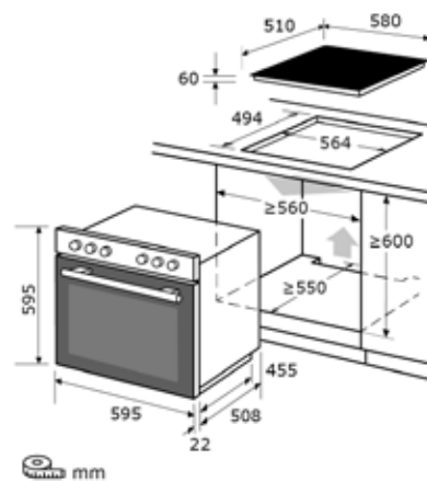
Einbauskizze zu EHE156-2.IU-Set
