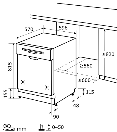
Einbauskizze zu EGSP6012-EB-030E inox
