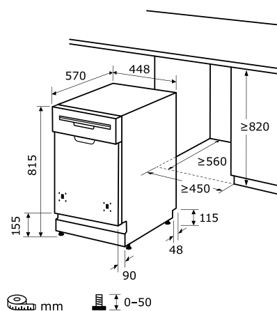
Einbauskizze zu EGSP2109-EB-030E inox
