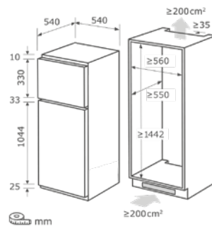
Einbauskizze zu EKGC265-40-040F
