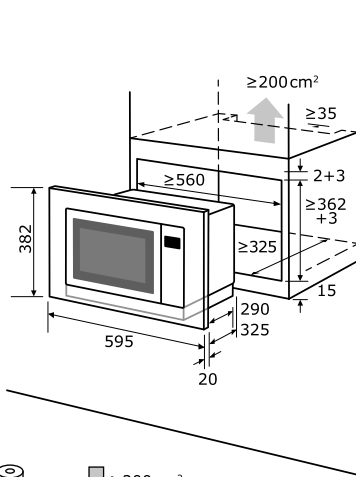
Einbauskizze zu EMW20-DG-020 inox | schwarz & EMW 20.1 G
