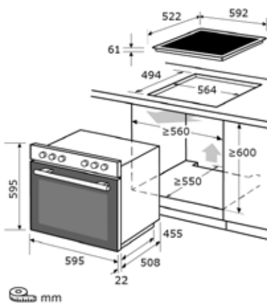
Einbauskizze zu EHE157-2URBZ-Set
