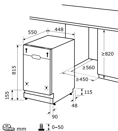
Einbauskizze zu EGSP9410-E-030D inox
