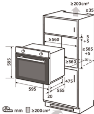
Einbauskizze zu EBEP697-H-030 schwarz
