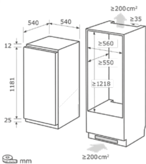
Einbauskizze zu EKS201-V-E-040F
