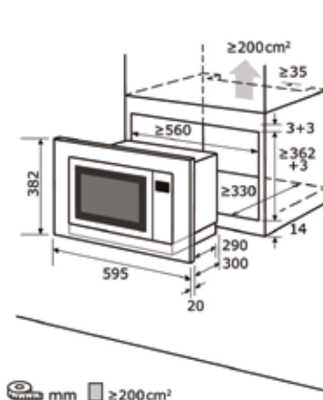
Einbauskizze zu EMW 1770-G-D-030 schwarz
