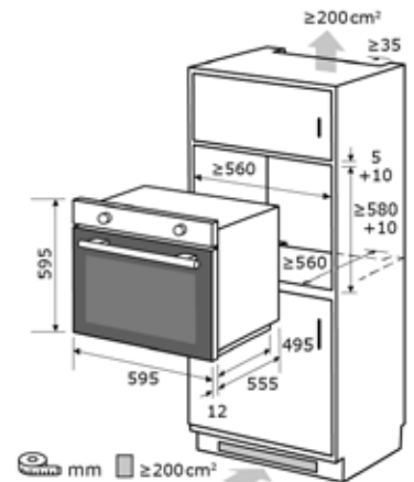
Einbauskizze zu EBE76-9-H-020 weiss | schwarz | inox
