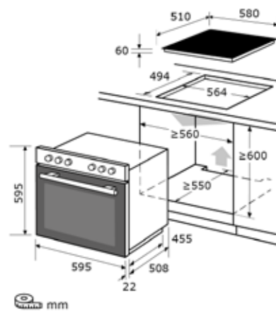
Einbauskizze zu EHE157-UBZ-020-Set schwarz
