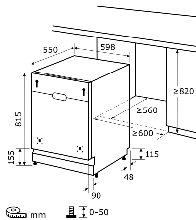
Einbauskizze zu EGSP2113-E-030E silber
