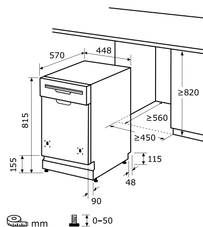
Einbauskizze zu EGSP1009-EB-030E inox
