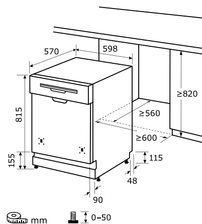
Einbauskizze zu EGSP9414-EB-030D inox
