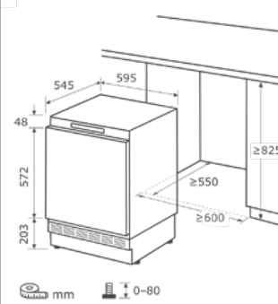
Einbauskizze zu UKS130-4-FE-010E
