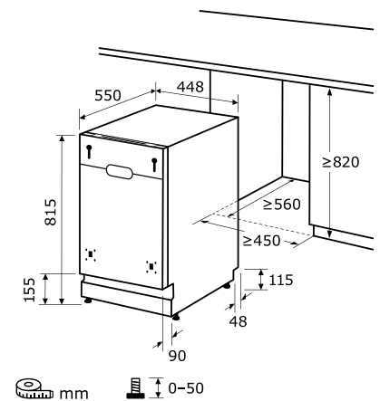
Einbauskizze zu EGSP2109-E-030E silber | EGSP1009-E-030E silber
