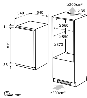
Einbauskizze zu EGS101-080F
