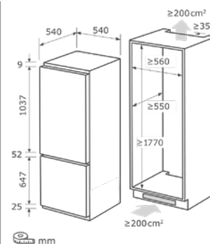
Einbauskizze zu EKGC270-70-E-040F
