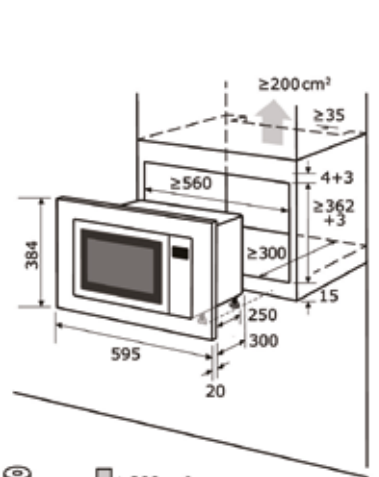
Einbauskizze zu EMW 19-7 G
