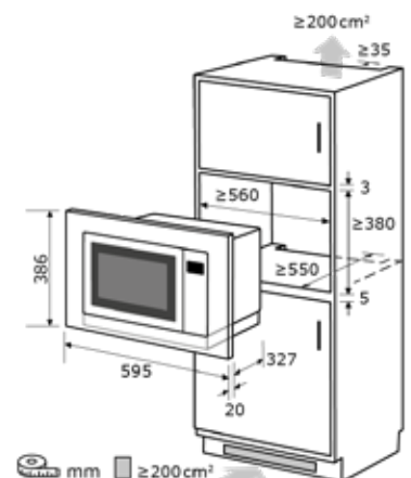
Einbauskizze zu EMW25-G-020 weiss | schwarz | inox
