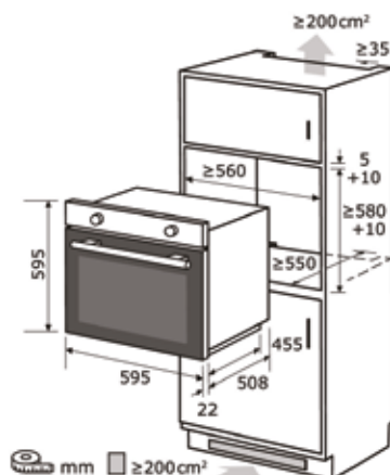
Einbauskizze zu EBE 555-2 U
