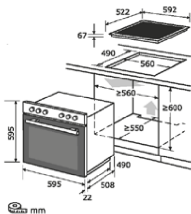
Einbauskizze zu EHE185-1.2-Set
