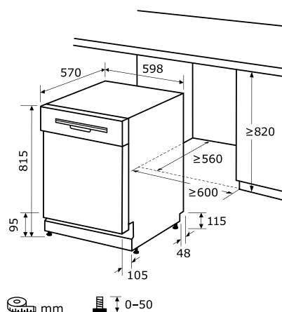
Einbauskizze zu EGSP9313-EF-030E inox
