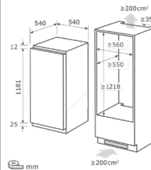
Einbauskizze zu EKS201-3-E-040F
