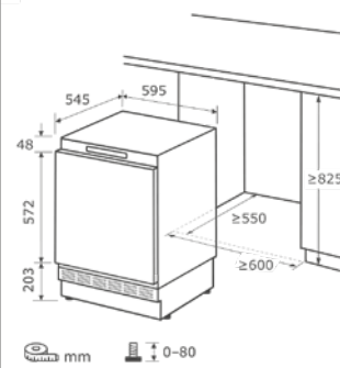
Einbauskizze zu UGS105-FE-010F
