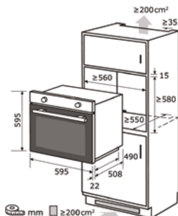
Einbauskizze zu EBE 555-1.1
