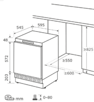
Einbauskizze zu UKS140-V-FE-010F
