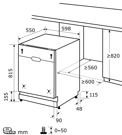
Einbauskizze zu EGSP1012-E-030E silber
