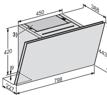
DAH2860 Skizze
