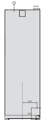
KWT4584E sw, Rioja, Installation (*Fußnote) (Skizze) *1) Ansicht von vorne, 2) Netzanschlussleitung, L = 2200 mm
