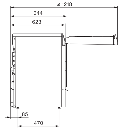
T2 mit Glastür, 17 Grad Blende, mit QuickPowerDry, Maße in mm
