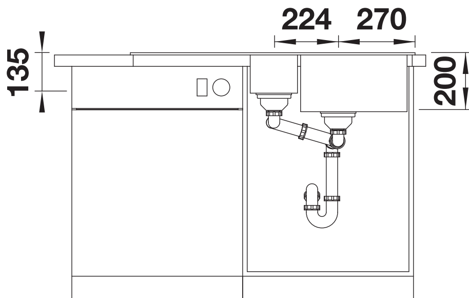
Frontansicht
