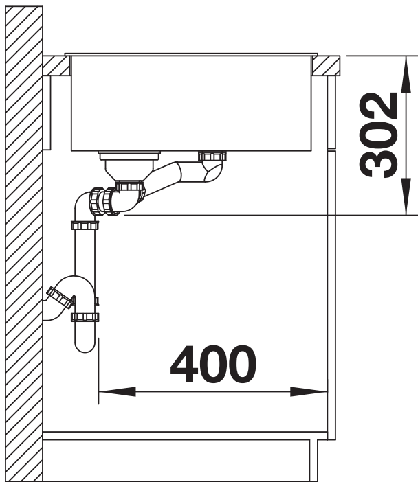
Seitenansicht
