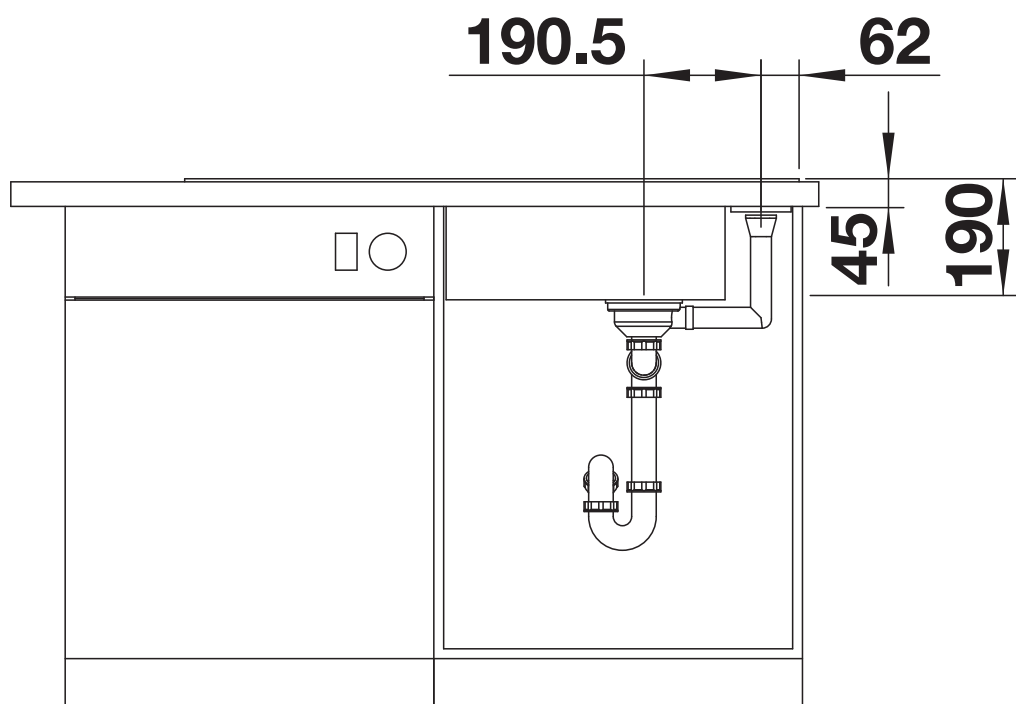
Frontansicht
