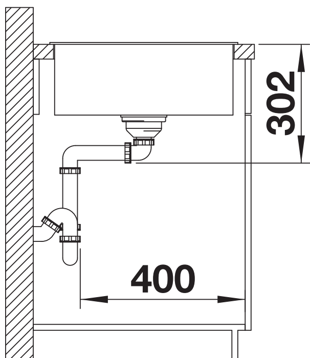
Seitenansicht
