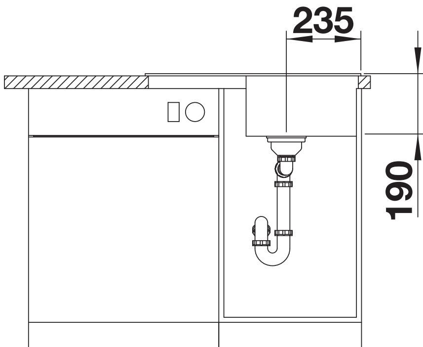
Frontansicht
