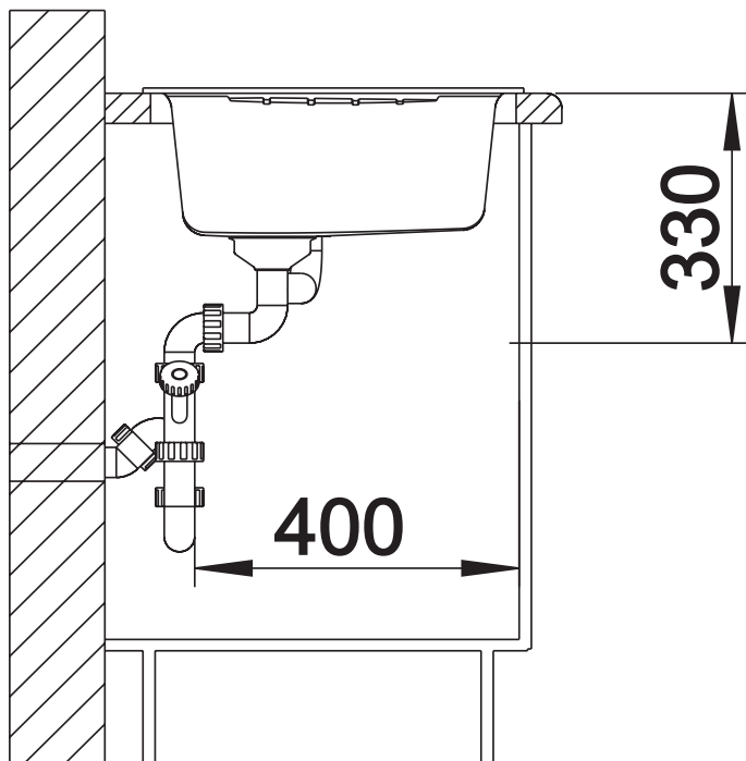
Seitenansicht
