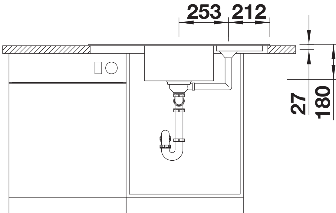
Frontansicht
