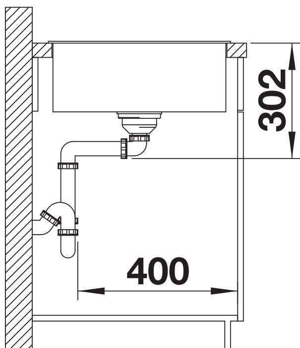
Seitenansicht
