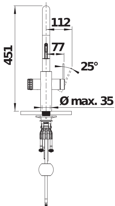
Seitenansicht Hebel
