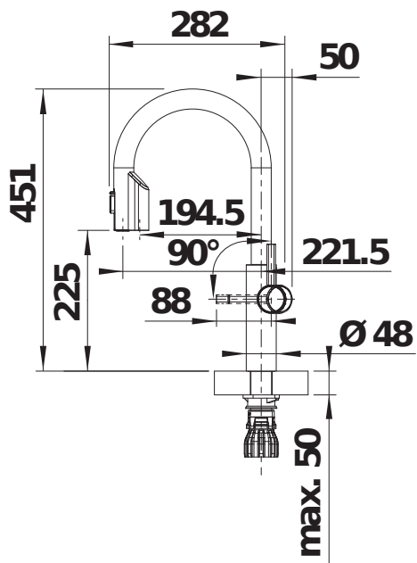
Seitenansicht
