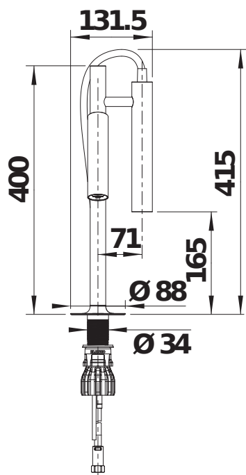
Seitenansicht Hebel
