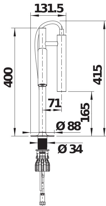
Seitenansicht Hebel
