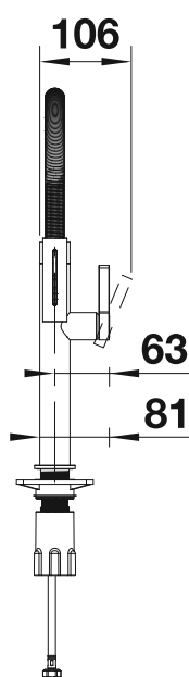
Seitenansicht Hebel
