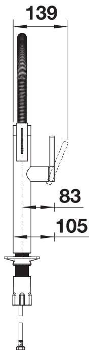
Seitenansicht Hebel
