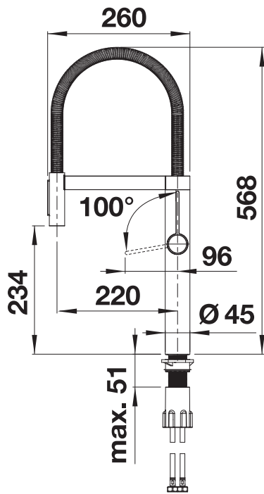
Seitenansicht
