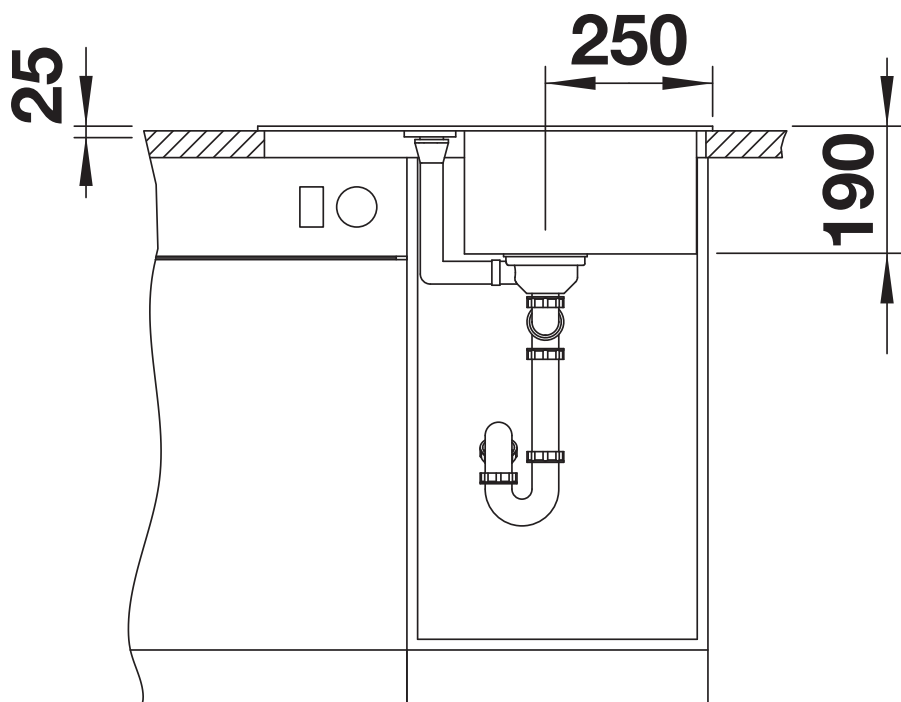
Frontansicht
