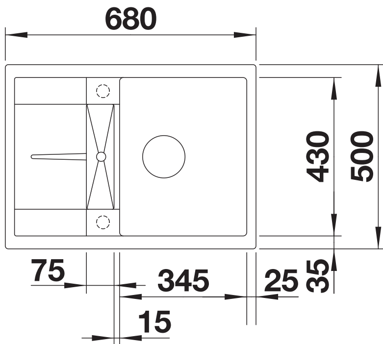
Aufsicht
