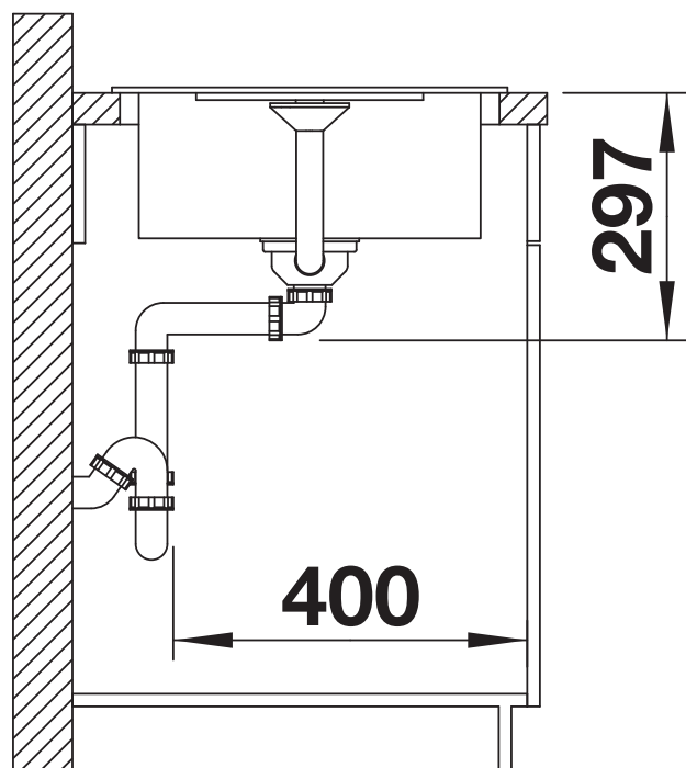
Seitenansicht
