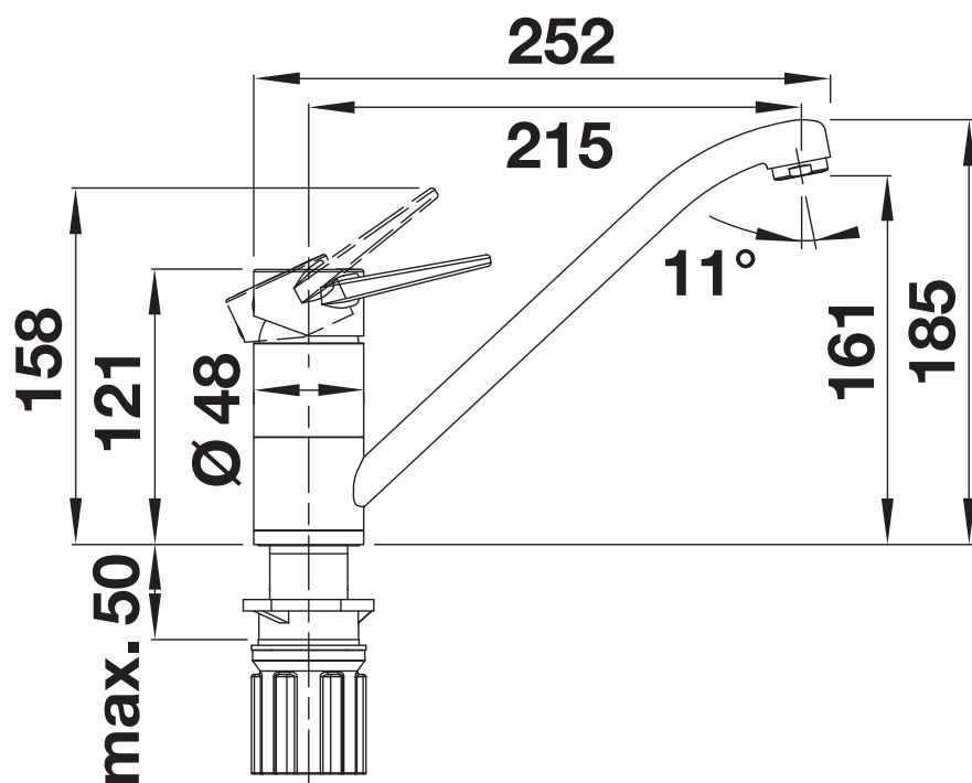
Seitenansicht
