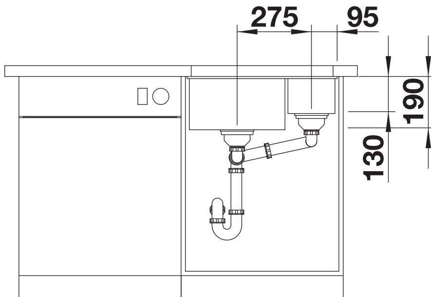
Frontansicht
