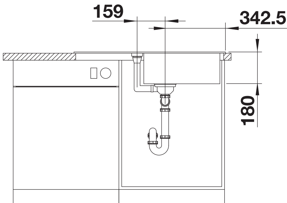
Frontansicht
