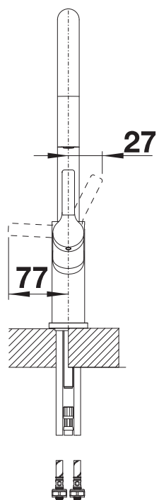
Seitenansicht Hebel
