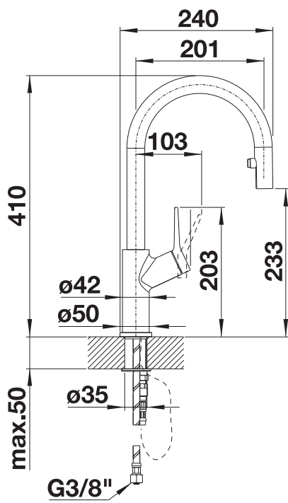
Seitenansicht
