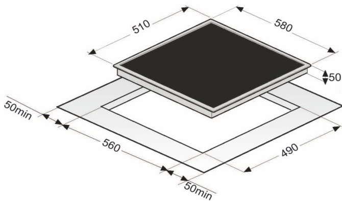
Einbauskizze
