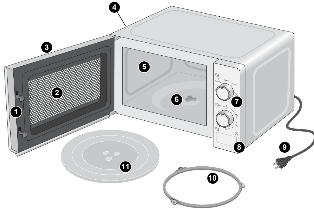
Abb. 1: Laitteen osat
