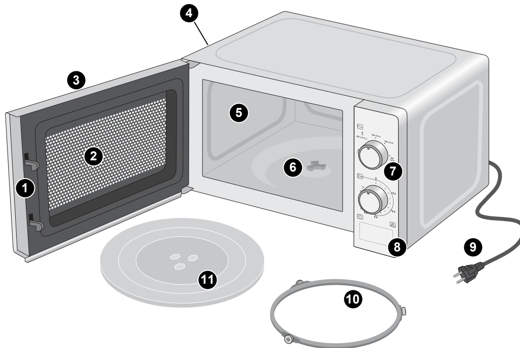
Abb. 1: Elementy urządzenia
