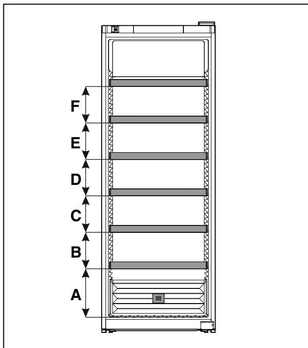
Fig. 18 Abstände Auflageroste
