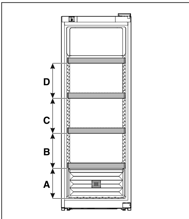
Fig. 14 Abstände Auflageroste
