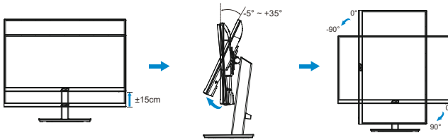
(Neigung)
