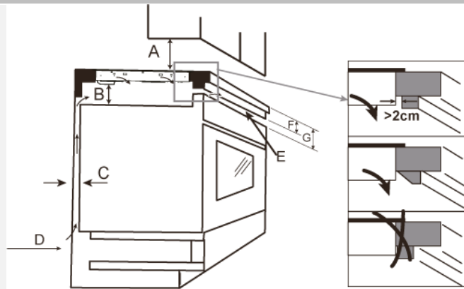
Grafik I: Einbauabstände B1= mit und ohne Wärmequelle
