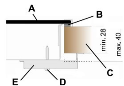
Abbildung 7 Querschnitt eingebauten Glaskeramikkochfeld
