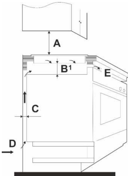
Abbildung 4 mit Wärmequelle
