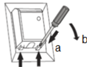
Abbildung 9 Netzanschlussdose
