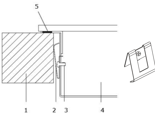
Abbildung 6 Glaskeramikkochfeld
