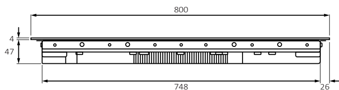
Vooraanzicht
