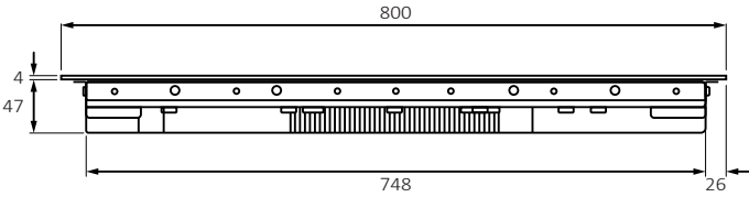
Vedere frontală
