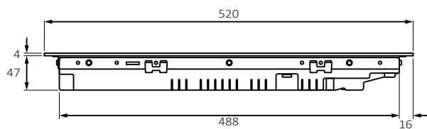
Zijaanzicht
