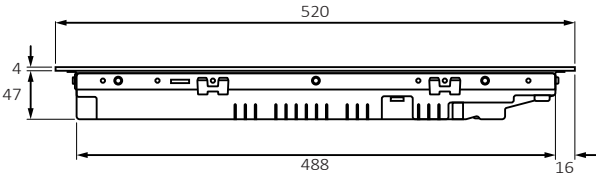
Vedere laterală
