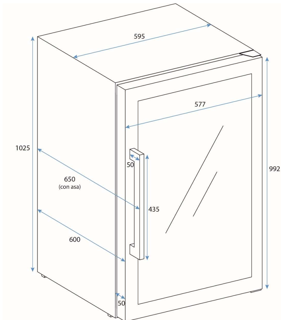
Figura: Dimemsionamiento
