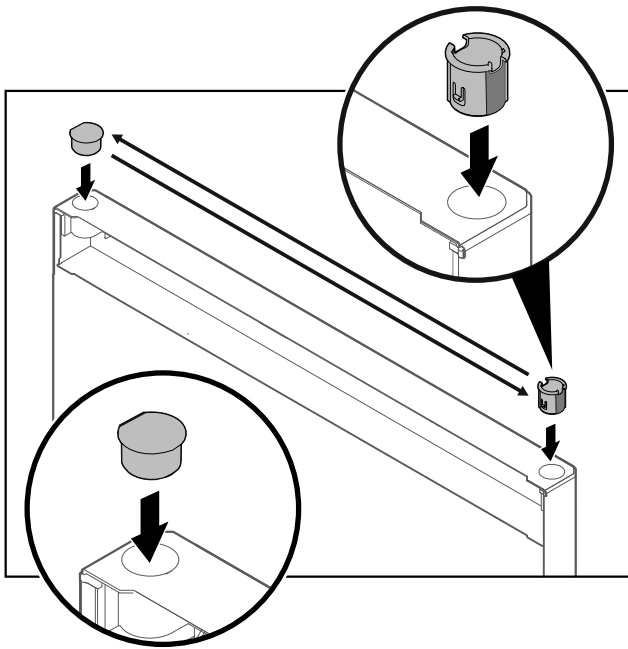
Fig. 23 Kühlteiltür
