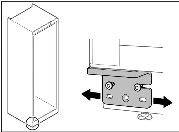
Fig. 67 Gefrierteil
