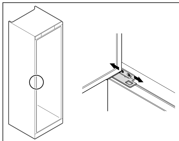
Fig. 65 Kühlteil
