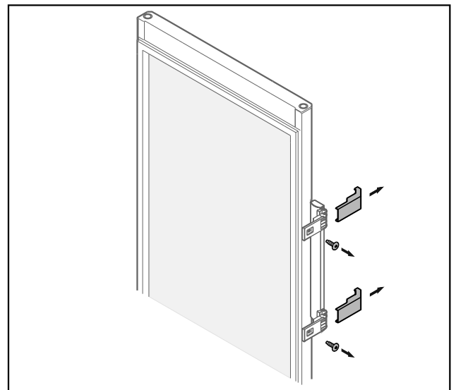
Fig. 31 Glastür*
