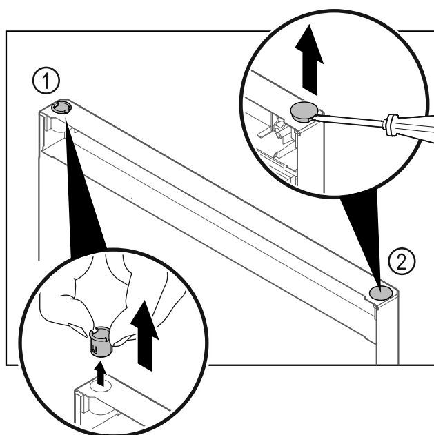
Fig. 22 Kühlteiltür
