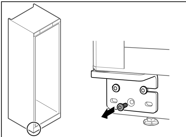
Fig. 66 Gefrierteil
