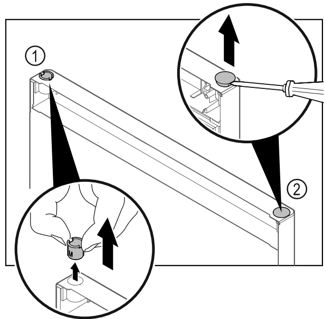
Fig. 35 Gefrierteiltür
