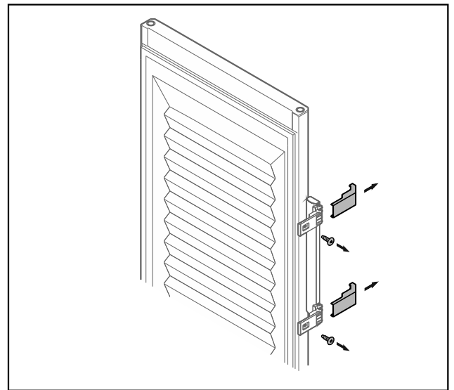
Fig. 30 Geschäumte Tür*
