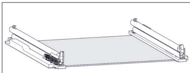
Fig. 124 Dämpfungseinheit
