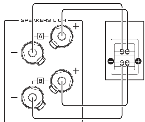
Achterpaneel van dit toestel
