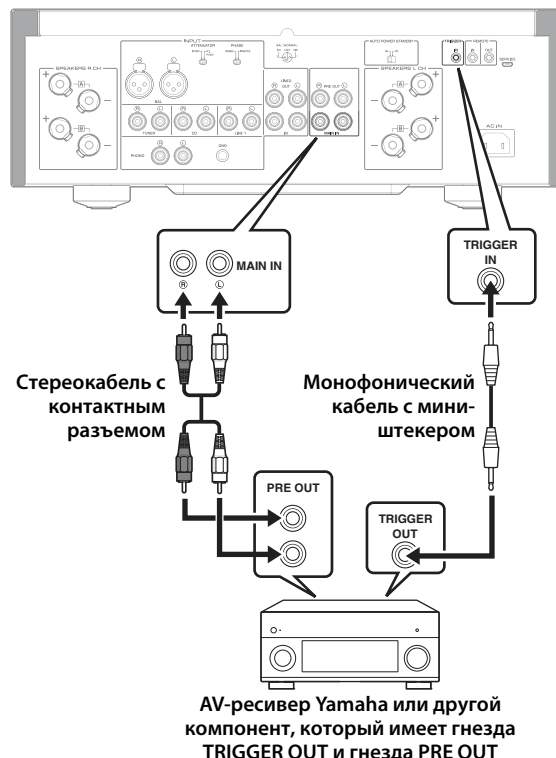
Задняя панель аппарата
