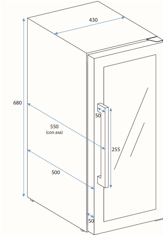
Figura: Dimensiamiento
