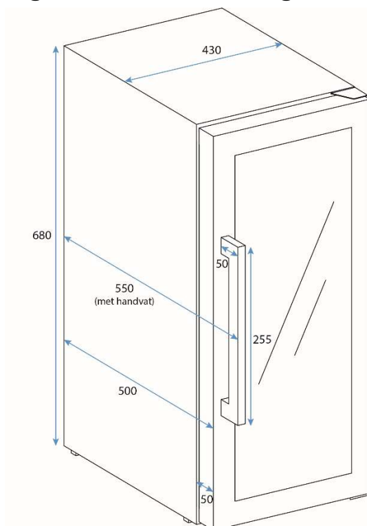
Figuur: Dimensionering
