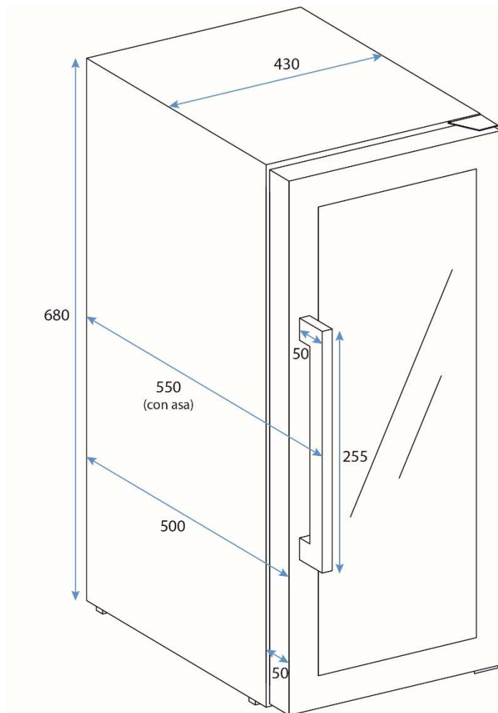
Figura: Dimemsionamiento
