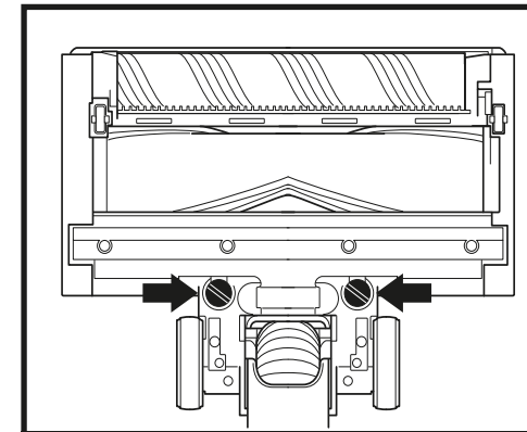
WISSER VERWIJDEREN
