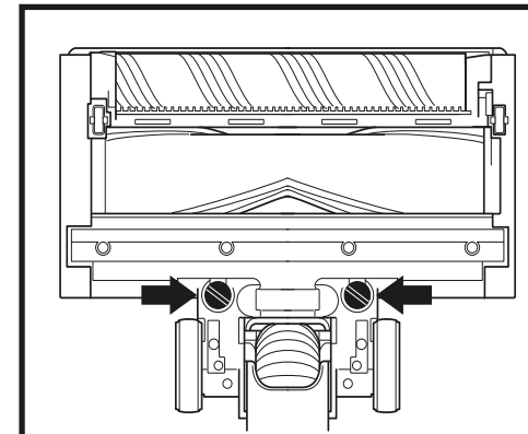
VEDENPURISTUSTELAN IRROTTAMINEN
