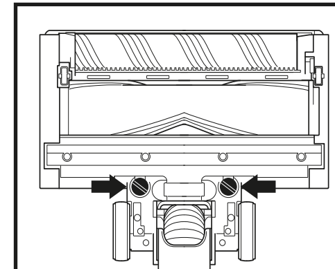
FJERNELSE AF SKRABER
