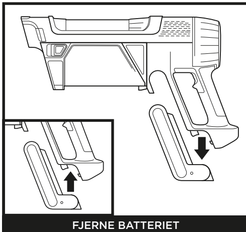
FJERNE BATTERIET
