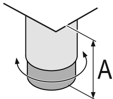
Fig. 14 Der Stellfuß ist von A = 115 mm (4 1/2 in) bis 175 mm (6 7/8 in) verstellbar.*
