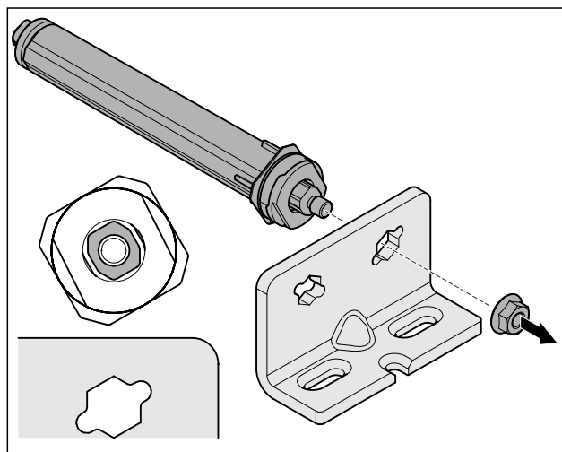
Fig. 29 Rechtsanschlag
