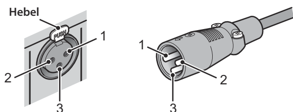
XLR-Buchse (weiblich)
