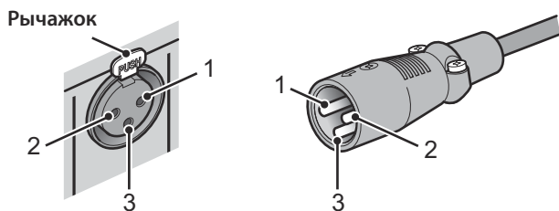
Гнездо XLR (гнездовое)
