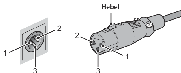
XLR-Buchse (männlich)
