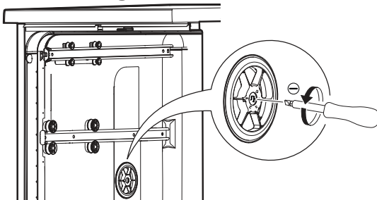
Abbildung 2: Mechanische Einstellgrafik
