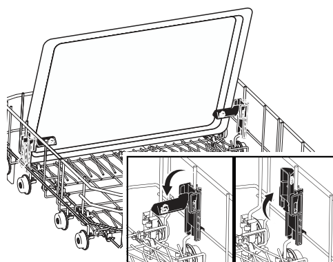
Abbildung 13: Backblech-Waschhalter
