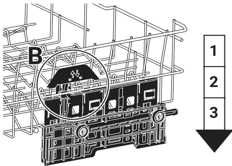
Abbildung 9: Verringerung der Stufen des oberen Korbs.
