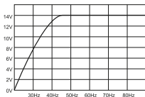
Bassleistung bei 50 Hz und 70 Hz mit Pufferkondensator
