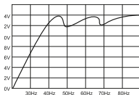
Bassleistung bei 50 Hz und 70 Hz ohne Pufferkondensator
