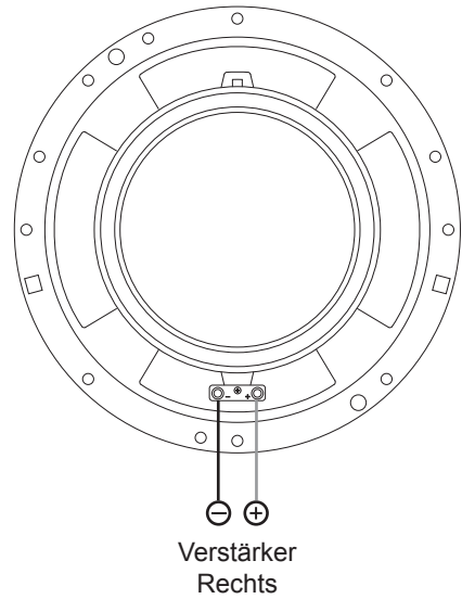
Tiefmitteltöner Rechts
