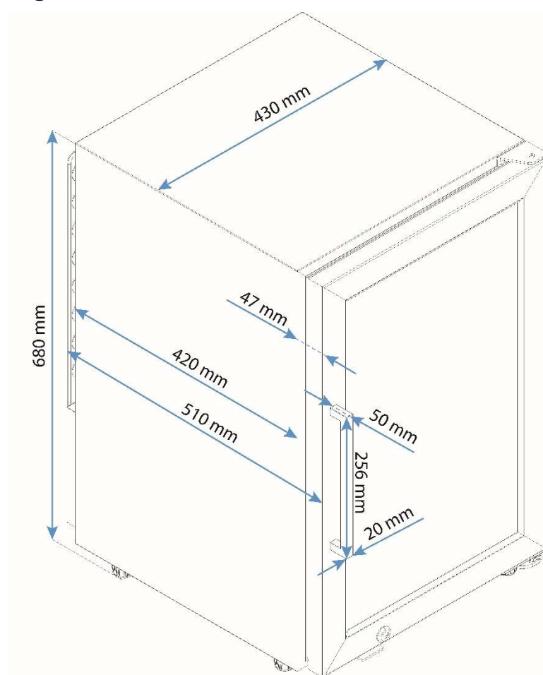
Figura: Dimensioamiento
