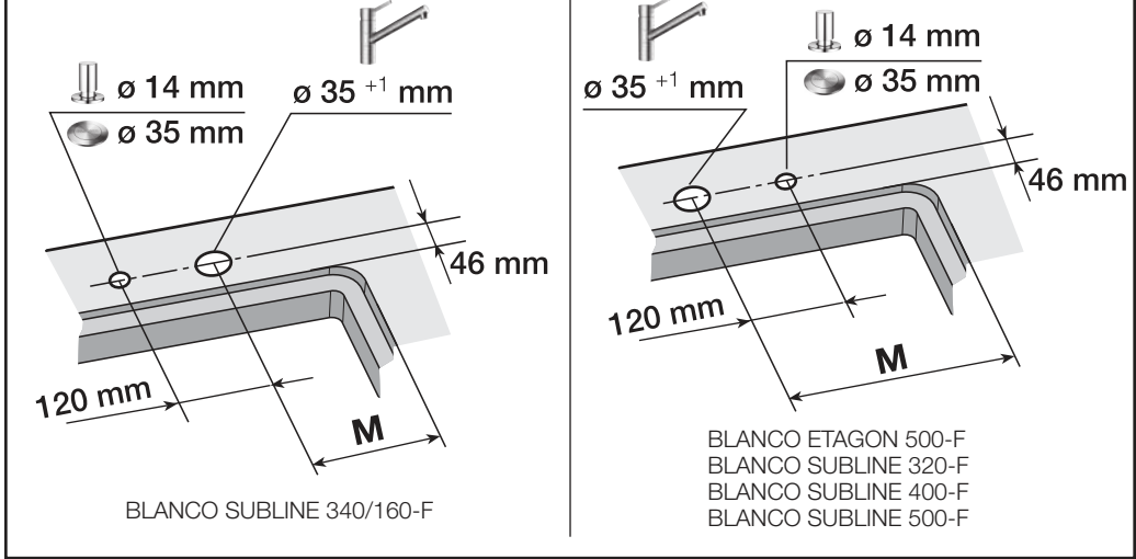
BLANCO SUBLINE 340/160-F
