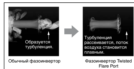
Турбулентия на обоих концах фазоинвертора создает шум
