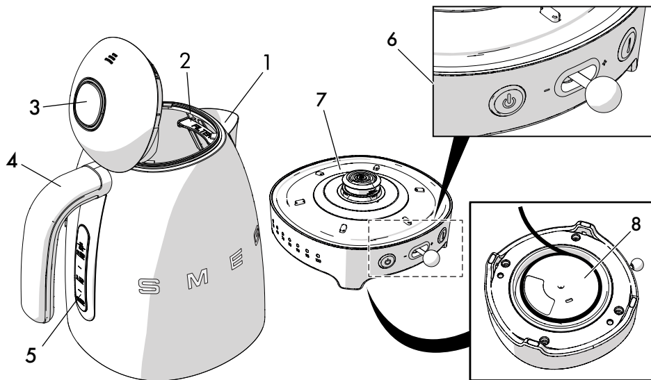
Modell KLF04 - Wasserkocher mit einstellbarer Temperatur
