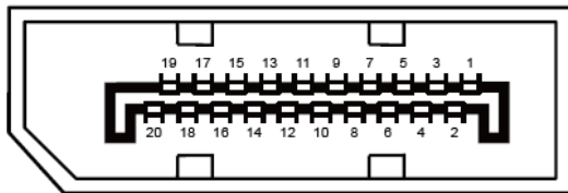
20-poliges Farbdisplay-Signalkabel
