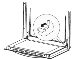
Abbildung 8 Backofentür 2
