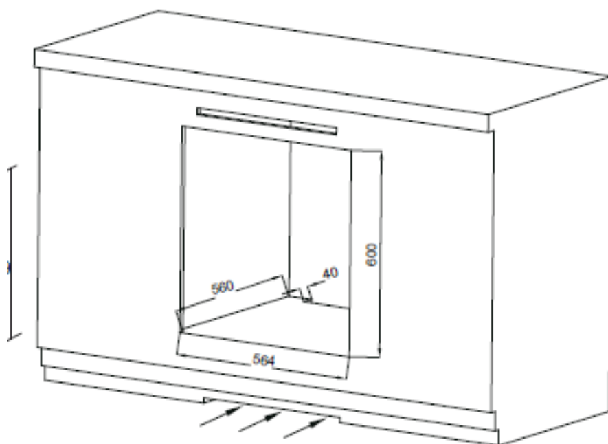
Abbildung 6 Einbaunische (A)
