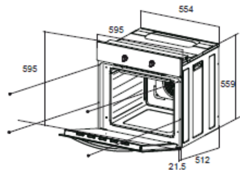
Abbildung 5 Gerätemasse
