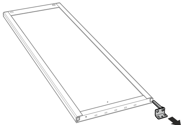
17. Scharnierwinkel herausziehen.
