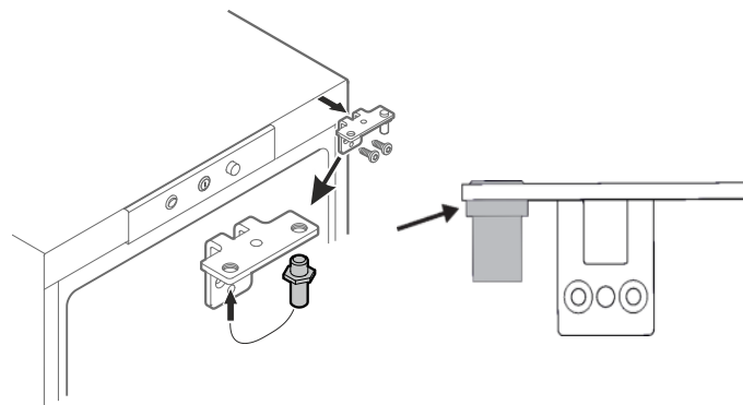
22. Scharnierwinkel abschrauben.
