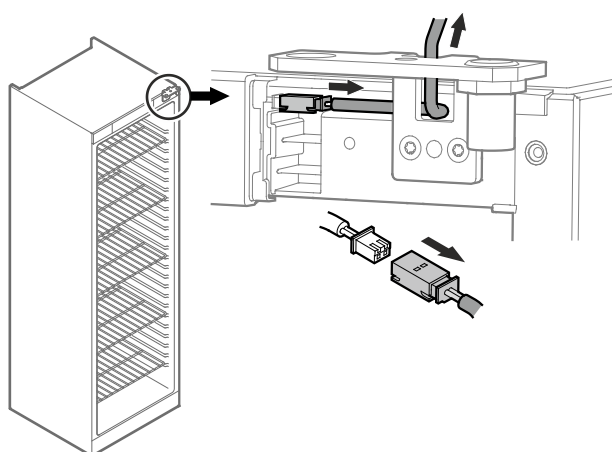
20. Stecker ausstecken.
