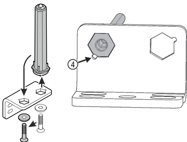
18. Bolzen im Scharnierwinkel umsetzen.
