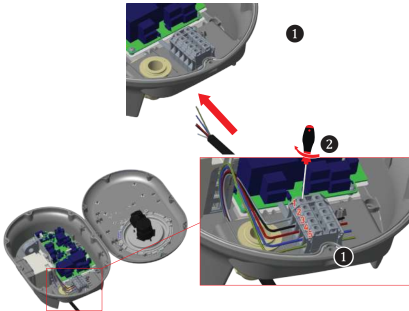
Abb.10: Netzanschluss 3-phasing
