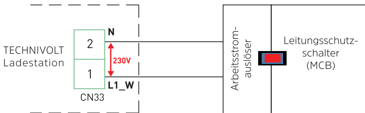
Abb.24: Anschluss Arbeitsstromauslöser
