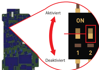
Abb.14: DIP-Schalter Nr. 2
