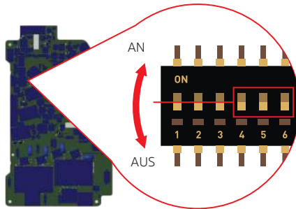
Abb.18:DIP-Schalter Nr. 4, 5, 6
